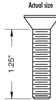
600-516-125
